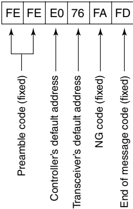
NG MESSAGE TO CONTROLLER
